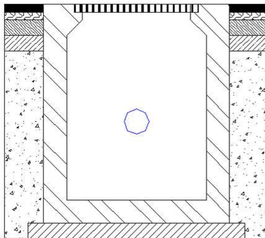
Σχήμα 4.6: Τομή φρεατίου υδροσυλλογής (το σχήμα είναι άνευ κλίμακας).
