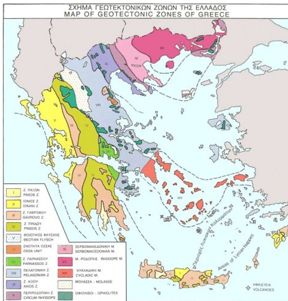
Σχήμα 3.1 Γεωτεκτονική θέση της περιοχής έρευνας
