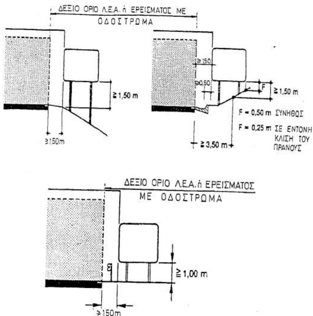
Σχήμα 1. Τοποθέτηση πλευρικών πλακιδίων κατά πλάτος της οδού.
